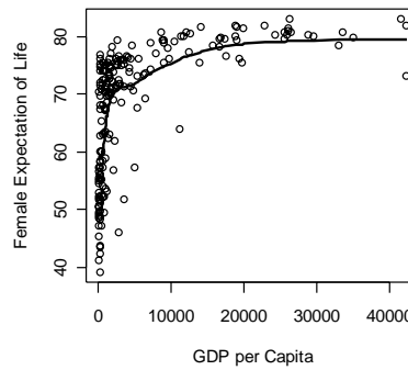
(d) Complete Kernel Estimate
